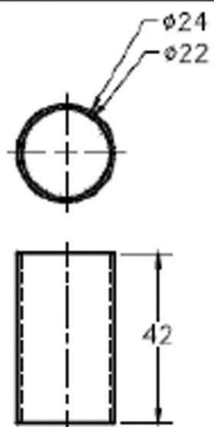
Rod Bush Upper
